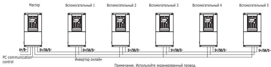
Рис. 19 Контурная схема
