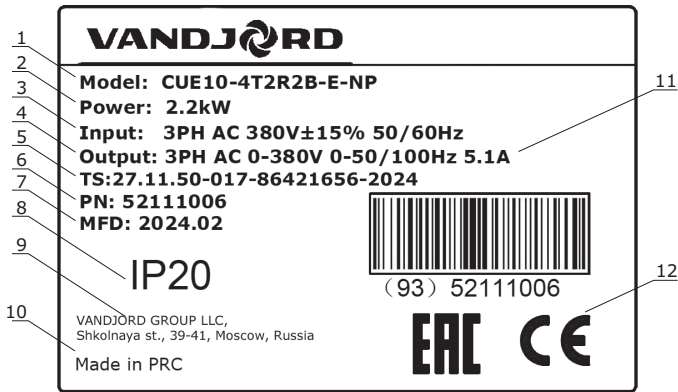
Рис. 1 Пример фирменной таблички
