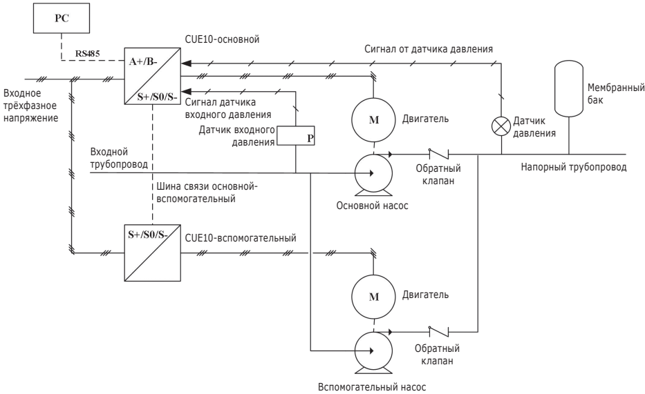
Рис. 23 Схема управления онлайн-системой
