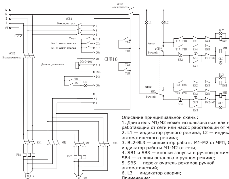
Рис. 24 Принципиальная схема 0,75–7,5 кВт
